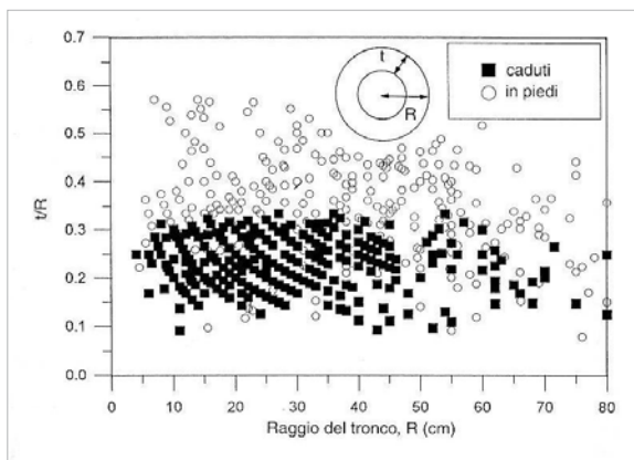
Figura 2 - Grafico t/R .
